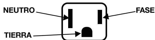
CONFIGURACIÓN DE RECEPTÁCULO NEMA 5-15R
