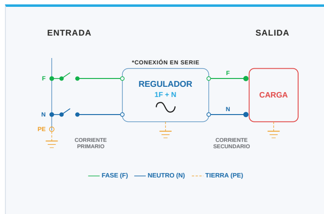
D - 001 Diagrama de conexión monofásica · 1F + N + Tierra Física
