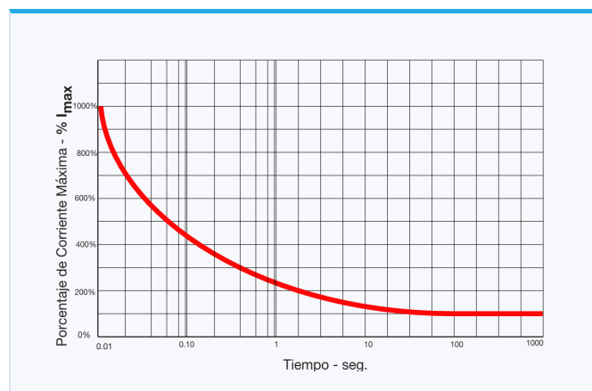
C-001 Sobrecarga · % I max vs tiempo (log seg)
